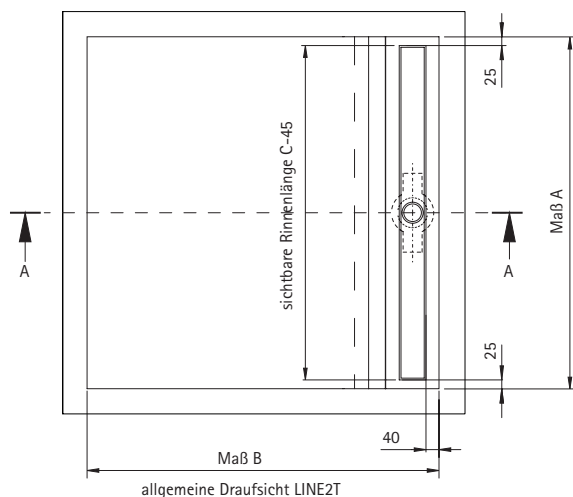
allgemeine Draufsicht LINE2T
