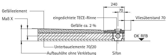
Schnitt A-A
